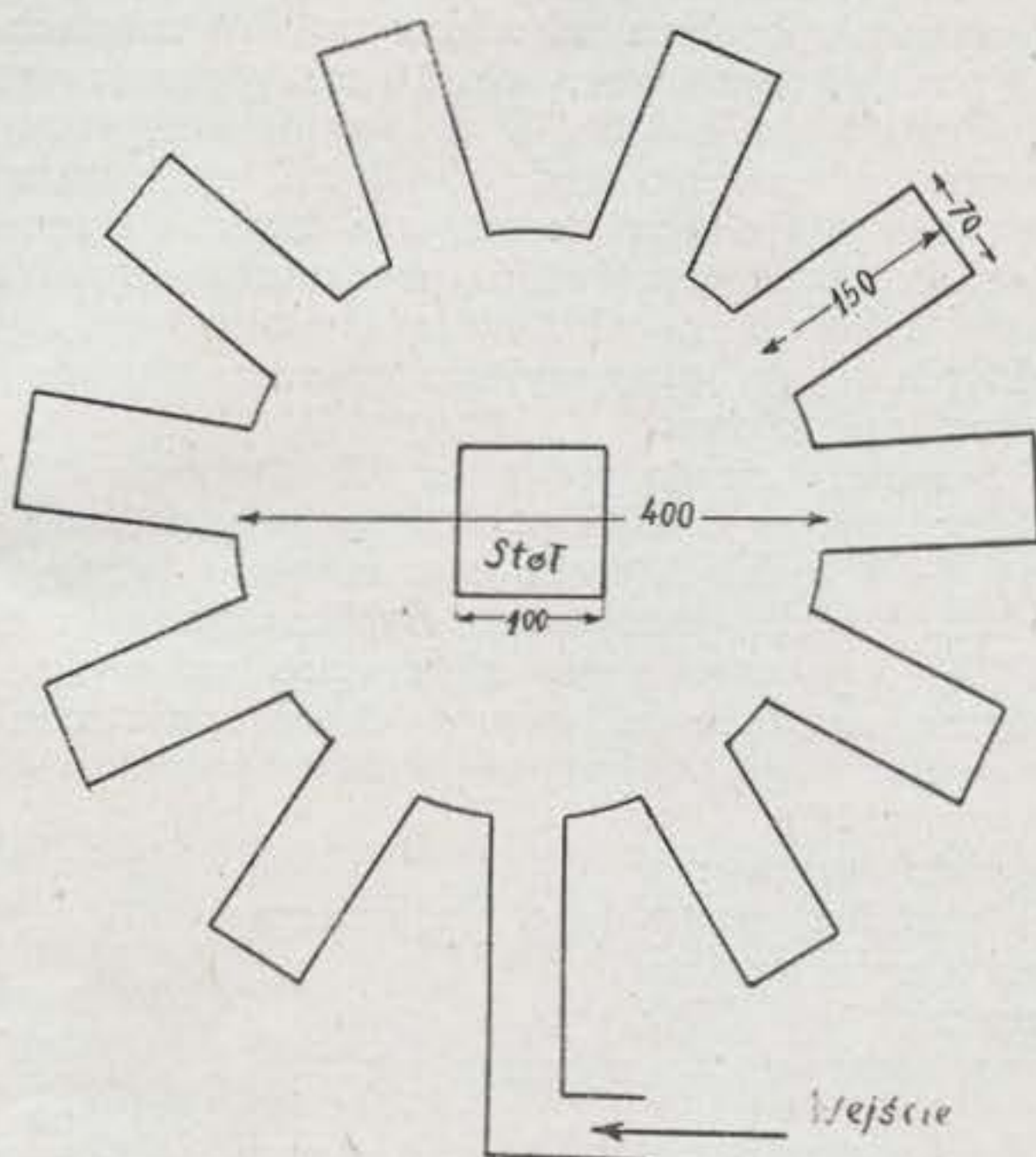
Schemat igloo 10-osobowego dla obozu stałego — rzut poziomy. Wymiary podane w centymetrach.
