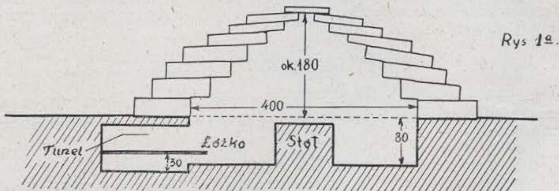
Schemat igloo 10-osobowego dla obozu stałego — przekrój pionowy. Wymiary podane w centymetrach.
