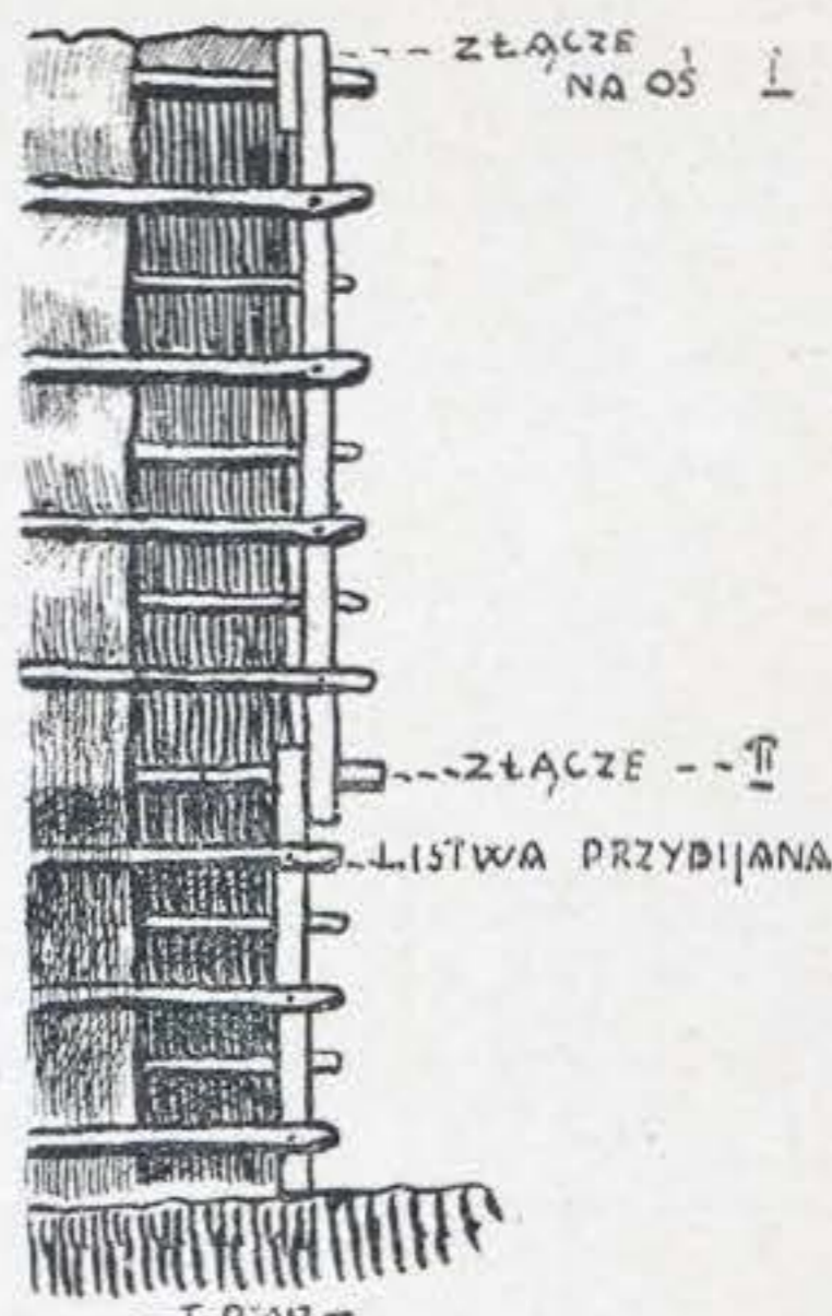
WIDOK BOCZNY SZALASKA (WIĄZANIA RAM). RYS 3
